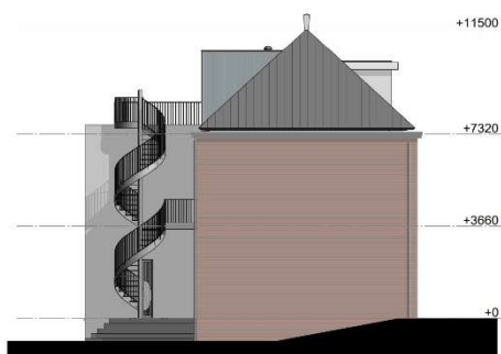
linker zijgevel
